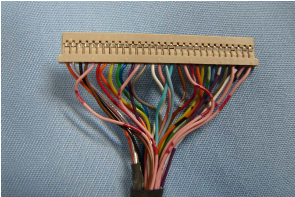
Foto 4. 2. Conector HIROSE
