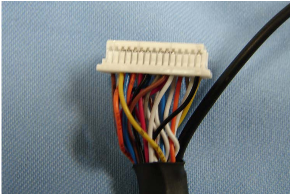
Foto 3. 3. Conector JST
